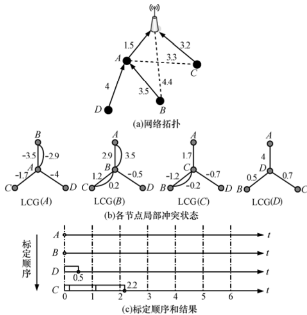
图 5 CT-TDMA 的执行过程 (实线表示逻辑链路, 虚线表示点到点之间的时延)
