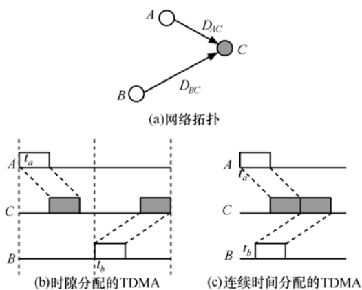
图 1 TDMA 不同策略下的发送时间的分配
